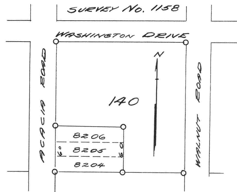
PLAT OF SURVEY OF LOTS 8204 TO 8206 OF LAKE COMO BEACH SUBD.
